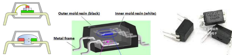
圖 6：光耦合器為將訊號發送端及接收端晶粒組合成之元件
